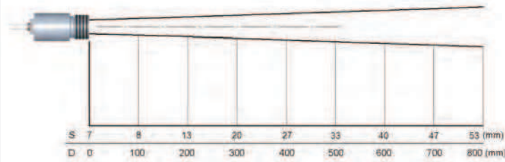
15:1 optics
